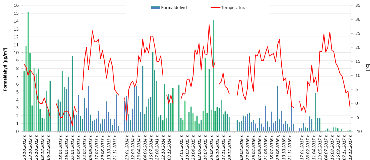
Rys. 2. Stężenia dobowe formaldehydu pomierzone w latach 2012-2017 na stacji w Żarach, przy ul. Szymanowskiego
