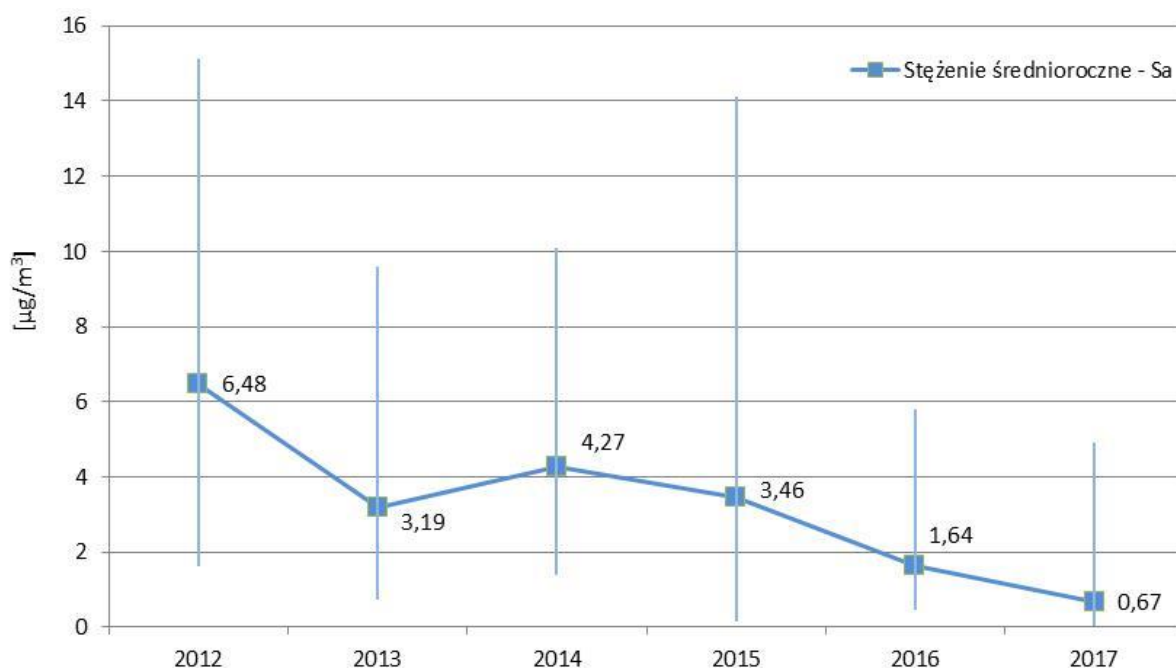
Rys. 1. Stężenia średnioroczne formaldehydu pomierzone w latach 2012-2017 na stacji w Żarach, przy ul. Szymanowskiego, wraz ze stężeniami dobowymi minimalnymi i maksymalnymi w danym roku
